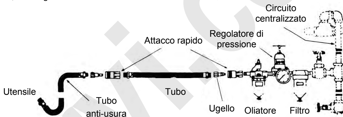
Figura 3 – Collegamento dell'alimentazione pneumatica.
