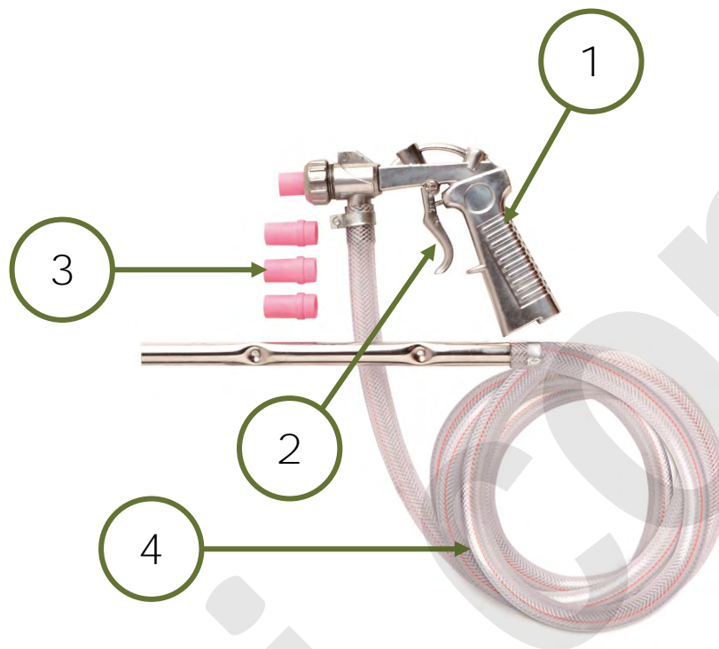
Figura 1 – Parti principali
